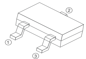
SOT-23-3L
