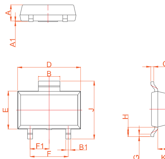
SOT-89-2L
