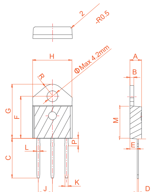
TO-3P Ins
