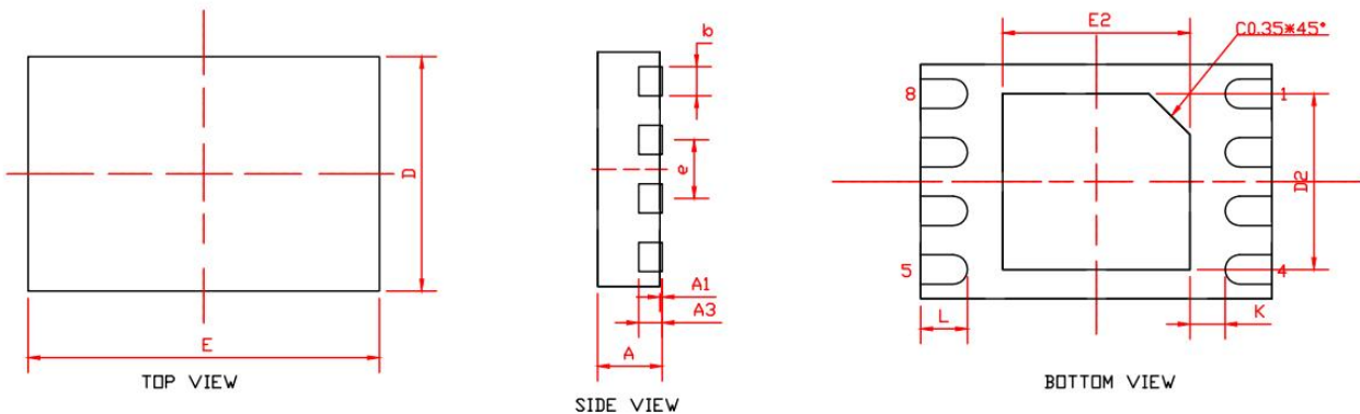
DFN2*3-8 封装信息
