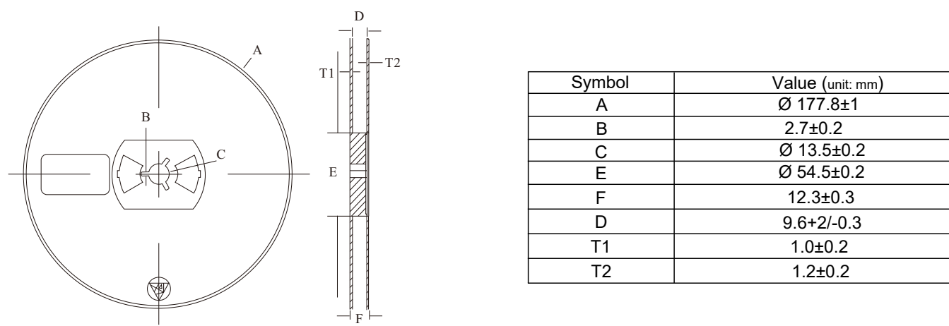
Reel (7")
