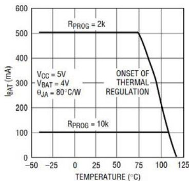
充电电流 vs 环境温度
