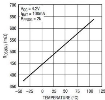
功率 MOS 开态电阻 vs 温度
