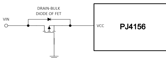
图 3：低损耗输入反向极性保护
