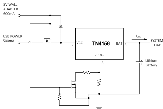
图 4：交流适配器与 USB 电源的组合
