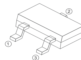
SOT-23-3L
