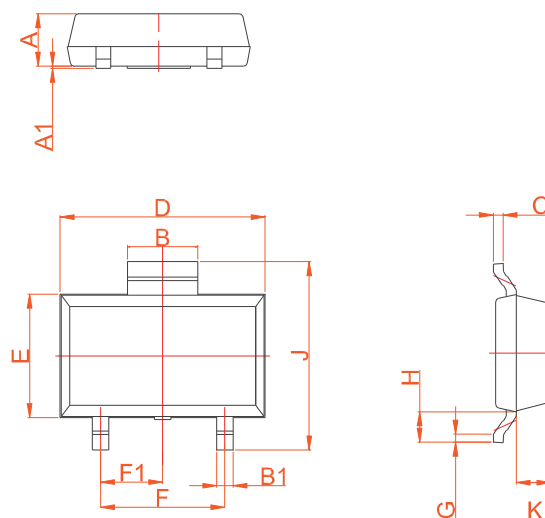
SOT-89-2L
